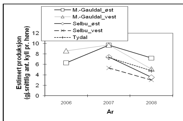
Figur 22: Produksjonsestimater fra taksering hos h.h.v. Hindsverk/Hindbjørgen-Holtsjøen og Soknedal grunneierlag i Midtre-Gauldal (2006-2008), Selbu fjellstyre og to utmarkslag i Selbu (2007-2008), samt Thomas Angells stiftelse i Tydal (2007-2008).
