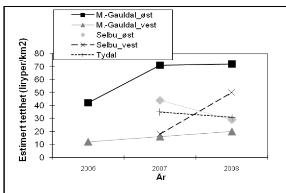
Figur 21: Tetthetsestimater etter bruk av Distance-metoden hos h.h.v. Hindsverk/ Hindbjørgen-Holtsjøen og Soknedal grunneierlag i Midtre-Gauldal (2006-2008), Selbu fjellstyre og to utmarkslag i Selbu (2007-2008), samt Thomas Angells stiftelse i Tydal (2007-2008).
