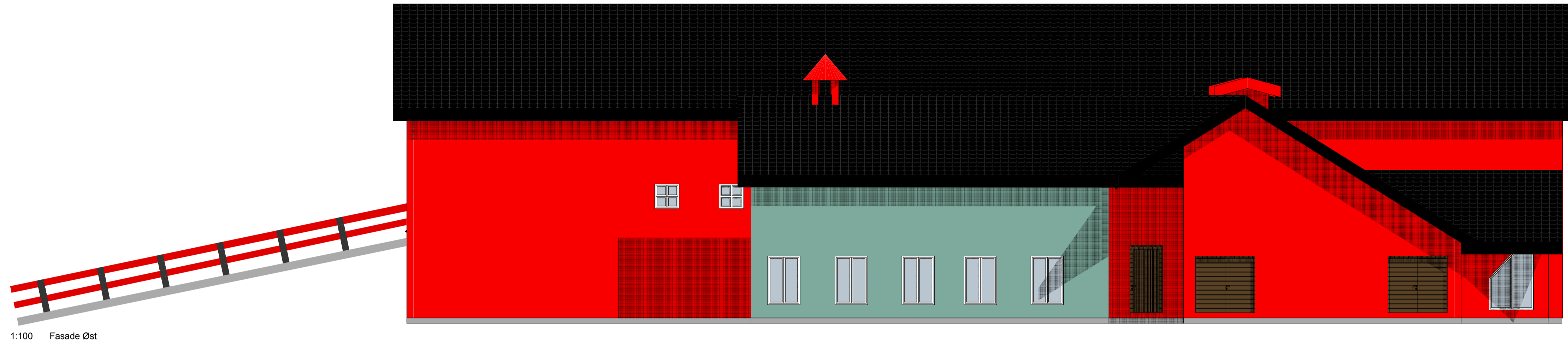
1:100 Fasade Øst
