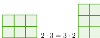
Figur 2.2.2.2: Den kommutative lov for multiplikasjon illustrert
